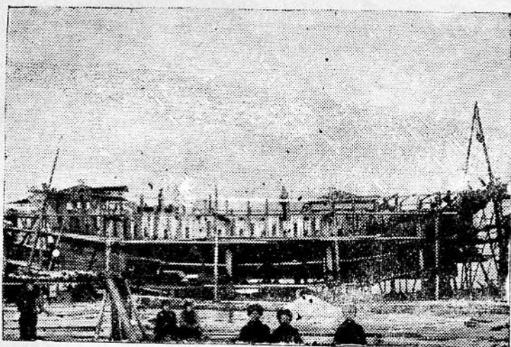
Сумский посад. Обшивка шпангоутов (ребер) вновь строящегося судна.
